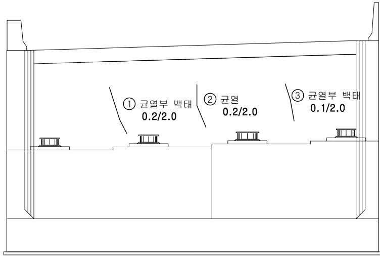
정면도
